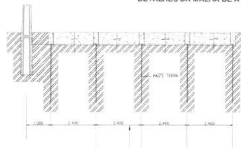
DETALHES DA MALHA DE ATERRAMENTO
