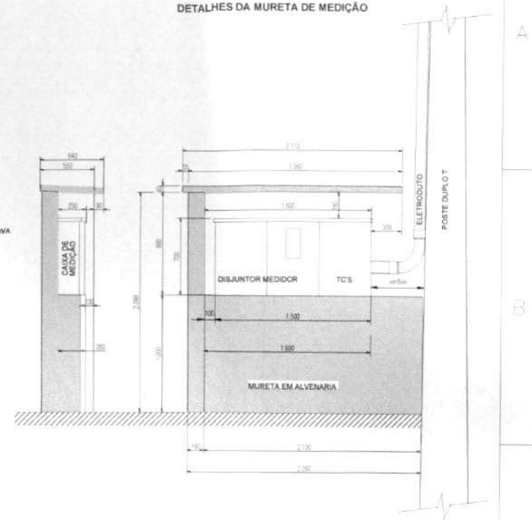
DETALHES DA MURETA DE MEDIÇÃO
